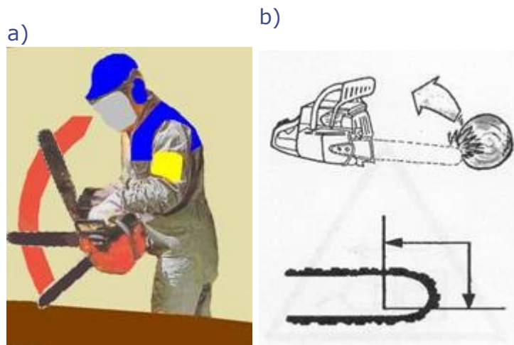
Rysunek 9. Odbicie pilarki: a) zjawisko odbicia, b) zetknięcie się górnej części końcówki prowadnicy z twardym przedmiotem
